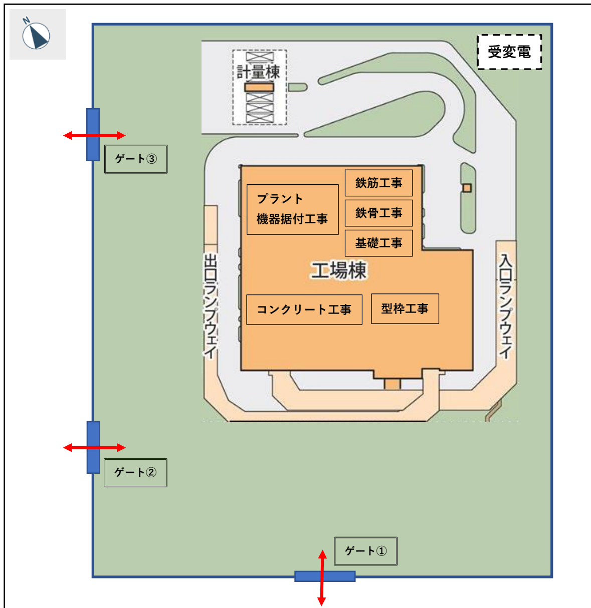
配置図
