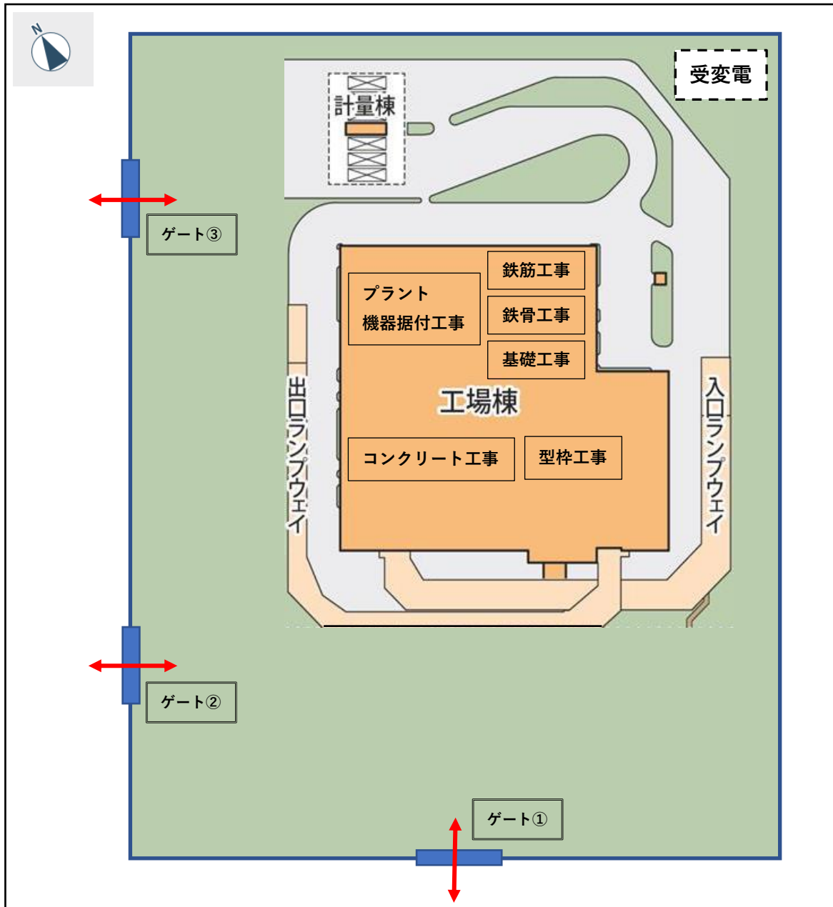
配置図
